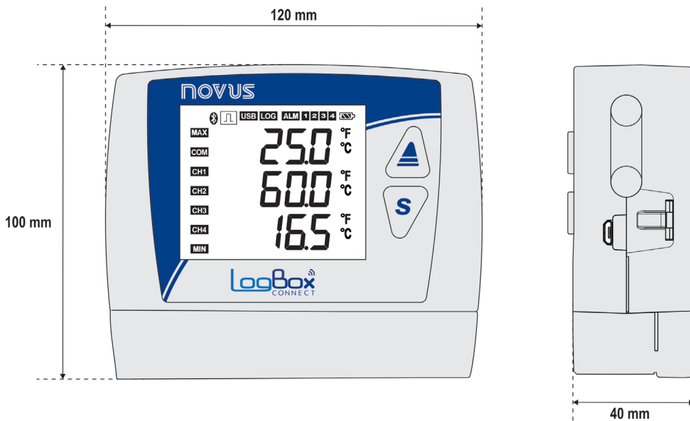
Fig. 45 – Dimensiones de LogBox-BLE
