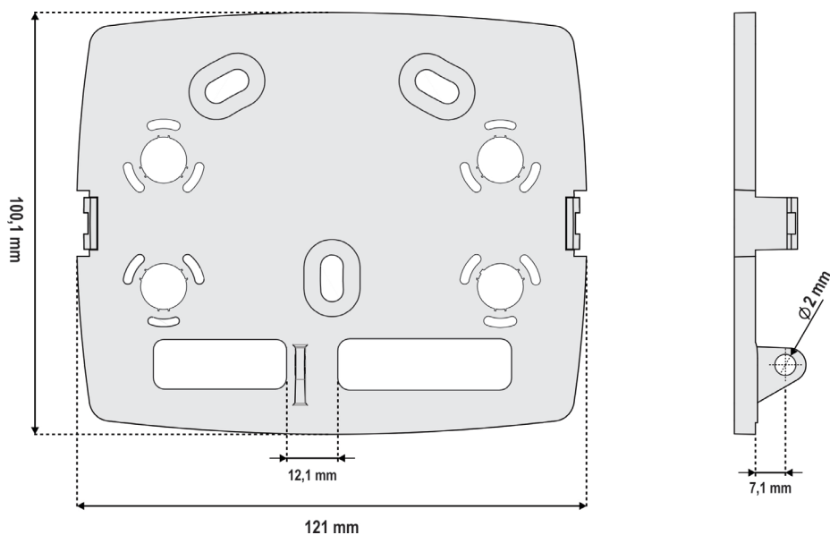
Fig. 40 – Soporte de fijación
