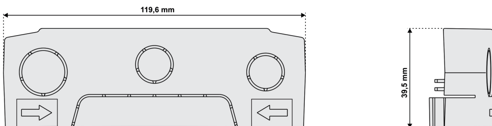
Fig. 42 – Dimensiones de la tapa de protección de las conexiones y cavidades separables
