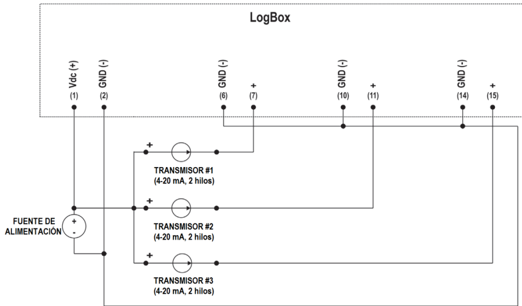
Fig. 49 – Ejemplo de conexión de transmisores alimentados por el loop
